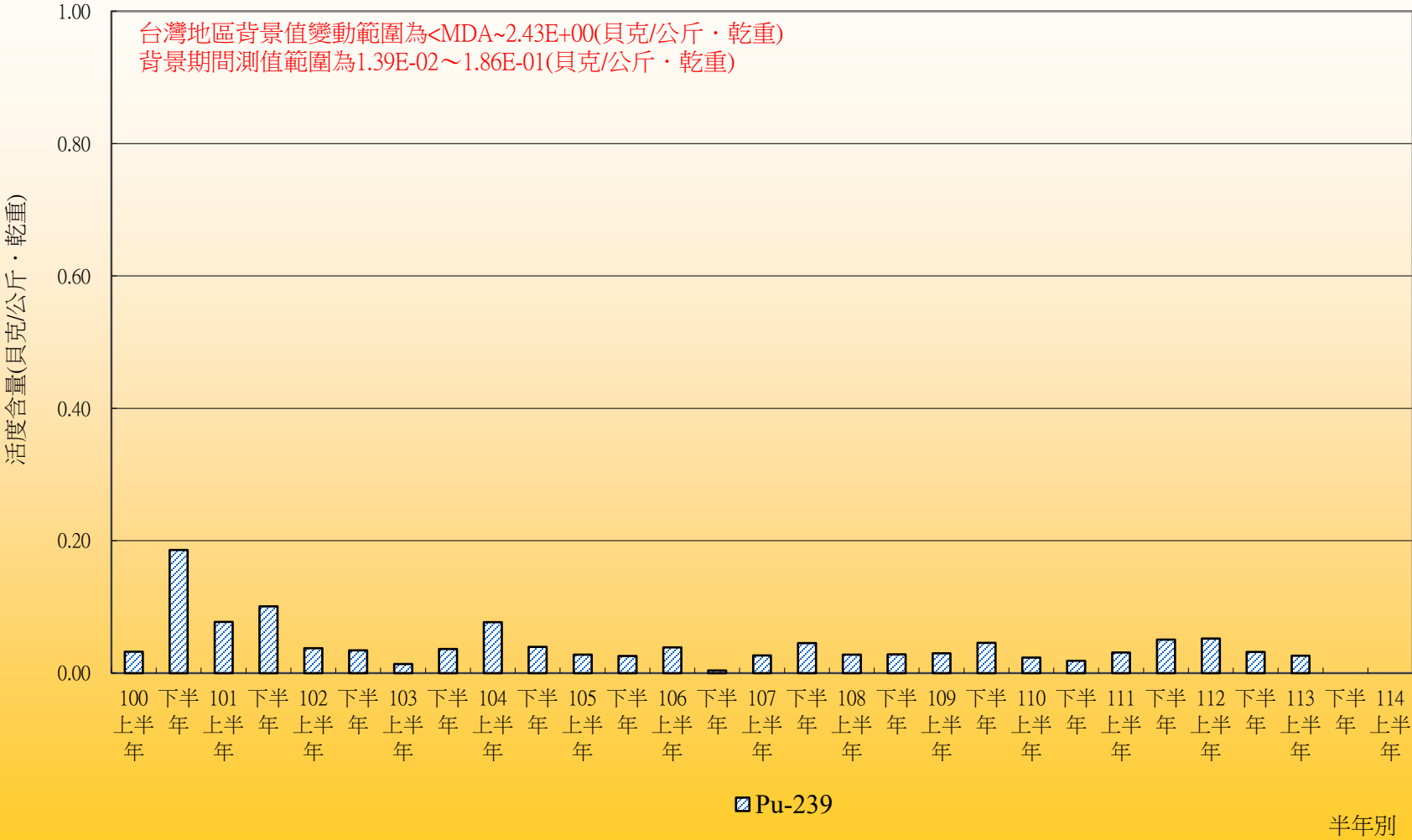
核二廠乾式貯存設施環境輻射監測 (土壤Pu-239)
